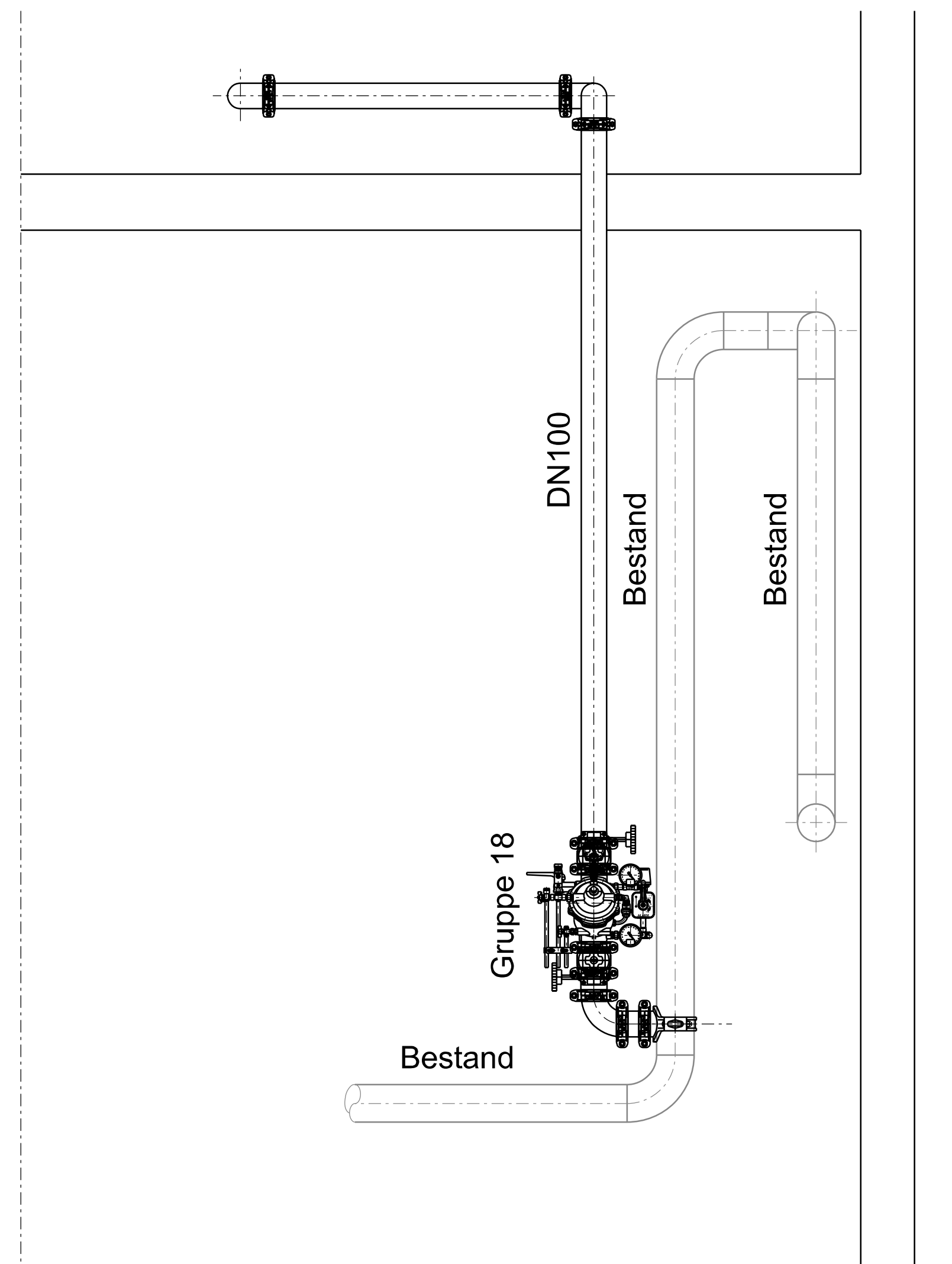
Ansicht Z
