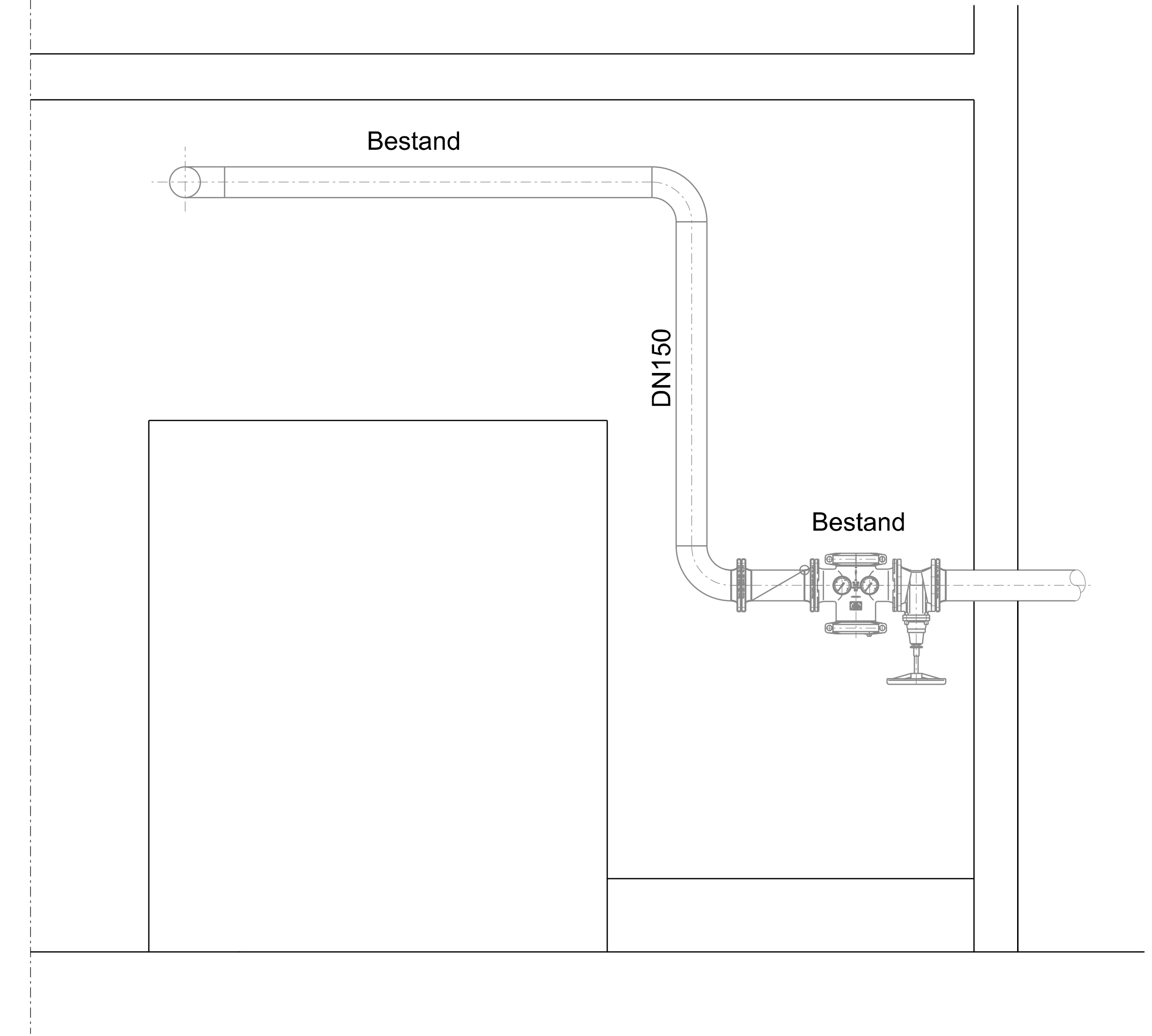
Ansicht Y
